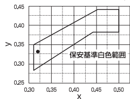
保安基準に規定されている色度範囲 '16年8月現在
