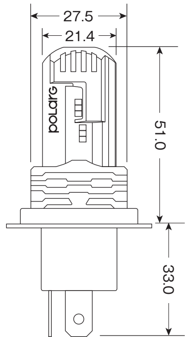
H4 TYPE
